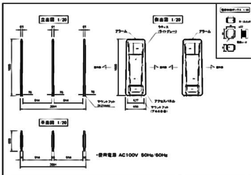
弊社作製2D図面
